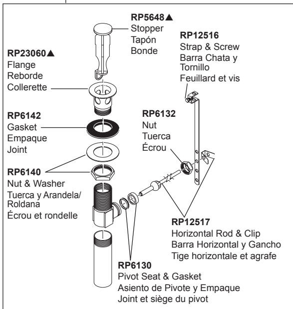
RP28653▲ Metal Pop-Up Assembly Less Lift Rod Ensamble de Metal del Desagüe Automático Sin la Barra de Alzar Renvoi mécanique en métal sans la tige de manoeuvre
