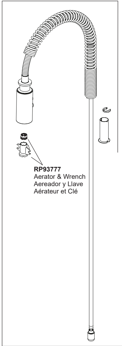
RP101728▲ Spring & Sprayer Assembly Ensemble de resorte y pulverizador Assemblage ressort et pulvérisateur
