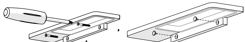
Installer la barre et les capuchons / Install the bar and the caps
