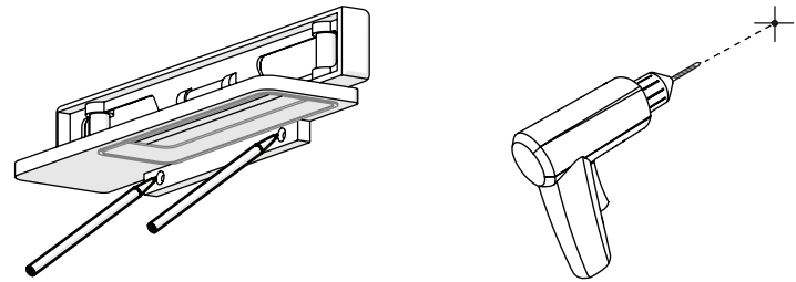
Marquer les points de perçage et percer / Mark the drilling locations and drill
